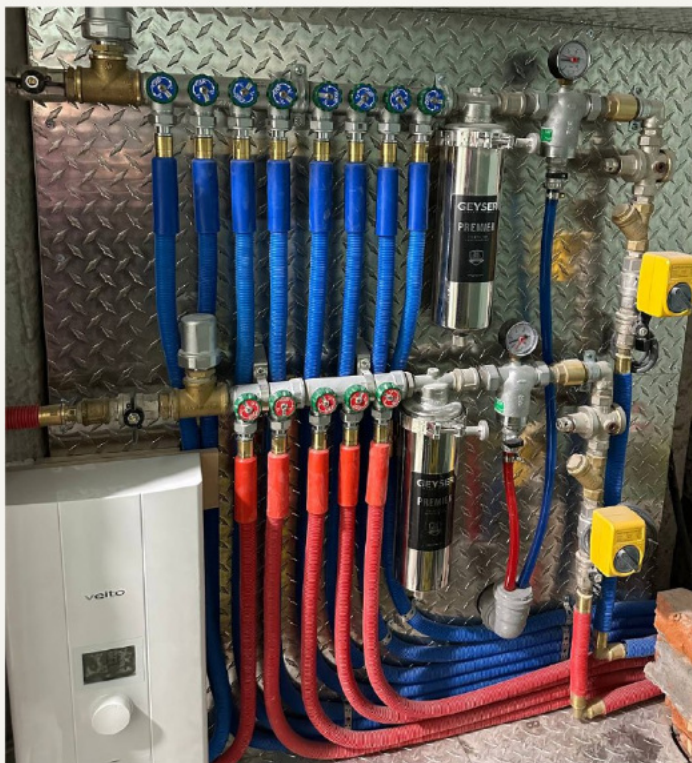
Водоснабжение
